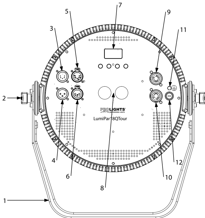
Pannello Posteriore
