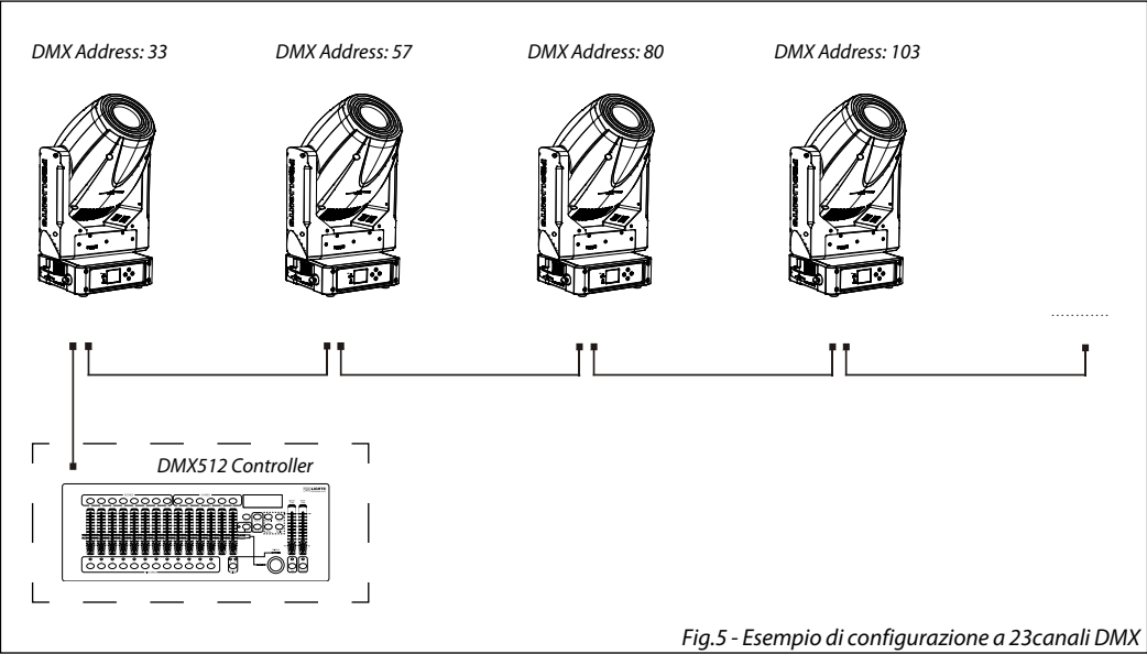
Fig.5 - Esempio di configurazione a 23canali DMX
