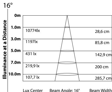
Diagramma di luminosità con alimentazione con cavo
